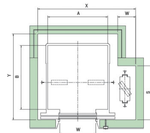
Mặt cắt ngang giếng thang hình vuông
