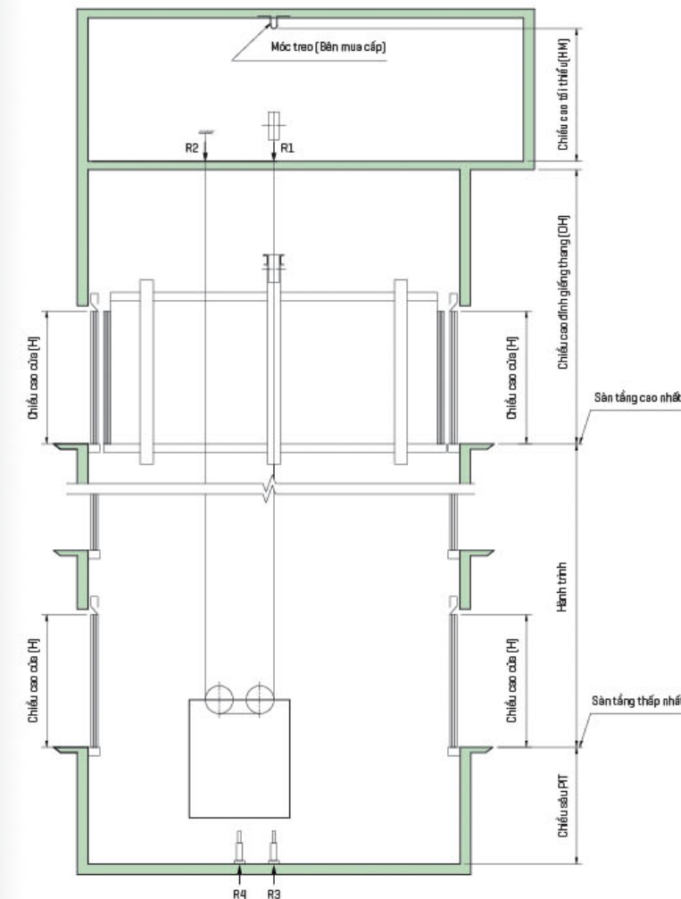
Mặt cắt đứng giếng thang
