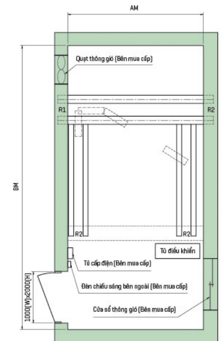
Mặt cắt ngang phòng máy
