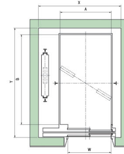
Mặt cắt ngang giếng thang
