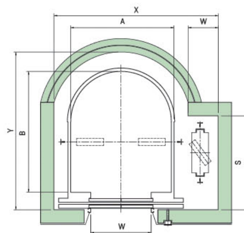
Mặt cắt ngang giếng thang hình bán nguyệt
