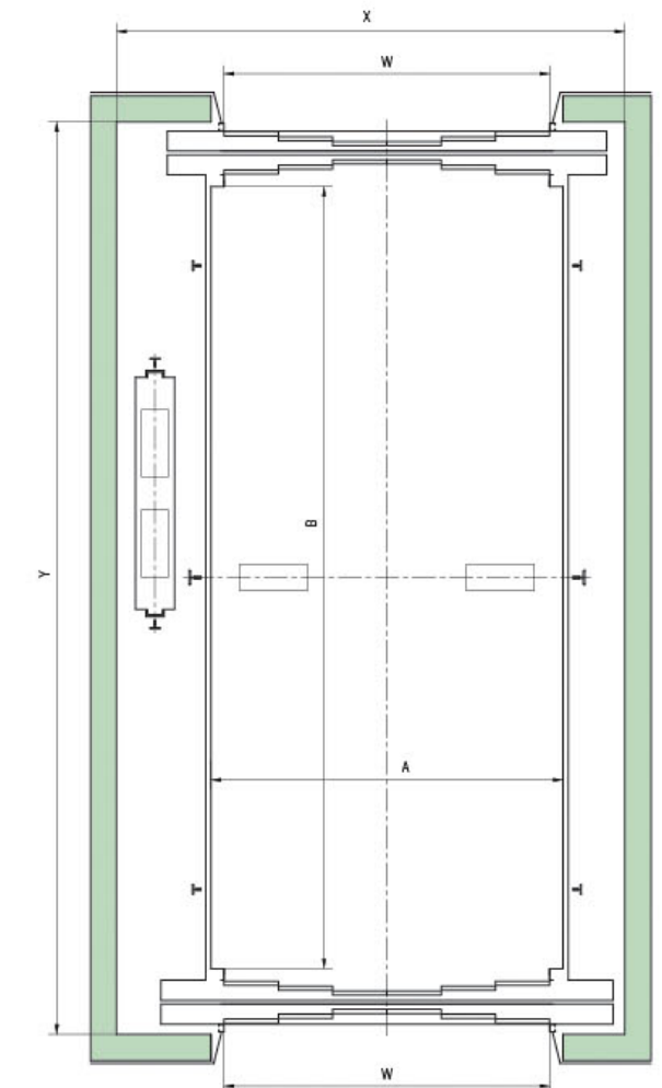
Mặt cắt ngang giếng thang
